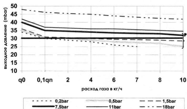
Характеристики регулятора LPZ 7 (30 mbar) NORMA EN 12864
